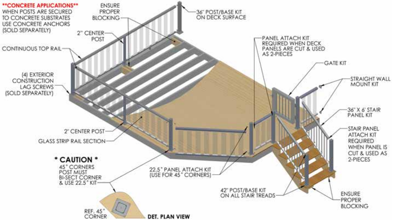
DET. PLAN VIEW
